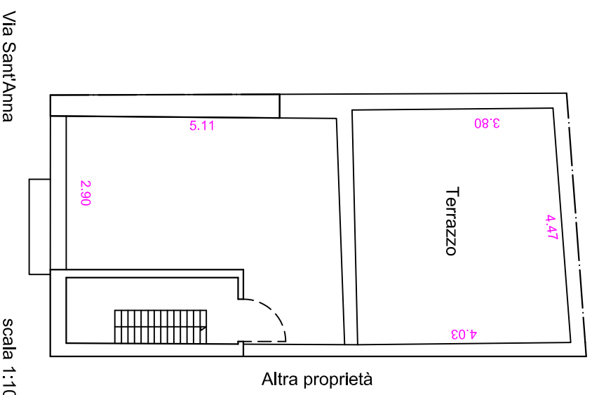
Pianta terrazzo
